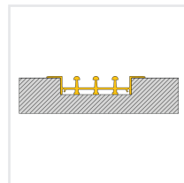
GUIDA INCASSATA A PAVIMENTO 3|4|5 VIE
