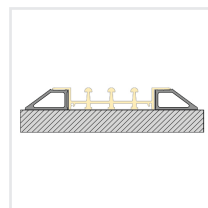
GUIDA A TERRA CON PROFILI SCIVOLO 3|4|5 VIE
